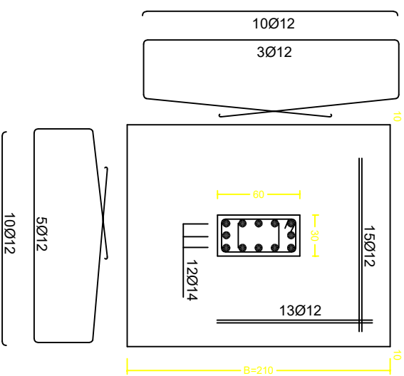
مقطع اساس اقواسي في العمود مع الاساس (C2, F2)
